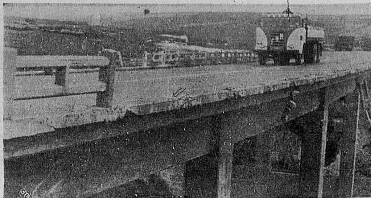
Há cinco meses um caminhão destruiu toda a parte lateral desta ponte, caindo e se destruindo completamente. Depois disso, mais outros dois carros tiveram o mesmo destino, com uma desvantagem: não havia proteção nenhuma. A ponte fica na Rodovia do Café, sobre o Rio dos Papagaios. São 48 metros de vão e, quando se vê ao longe a ponte, tem-se a impressão de que a estrada vai acabar ali.
