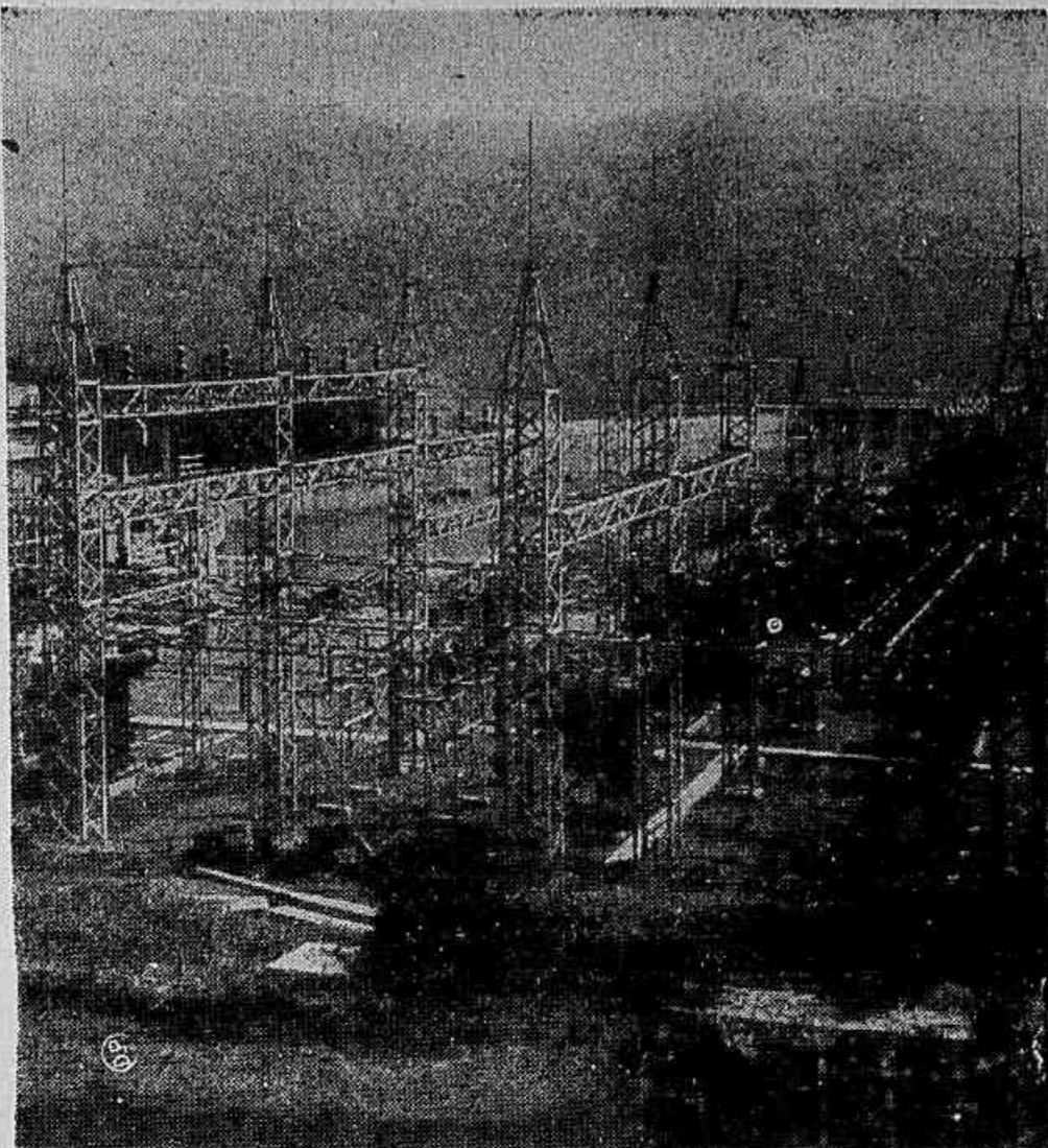
A subestação elevadora da Usina de Salto Grande do Iguaçu está situada à esquerda da Casa do Força, possuindo 5 transformadores elevadores. A alimentação dos centros de consumo será feita mediante três linhas de saída da subestação.
