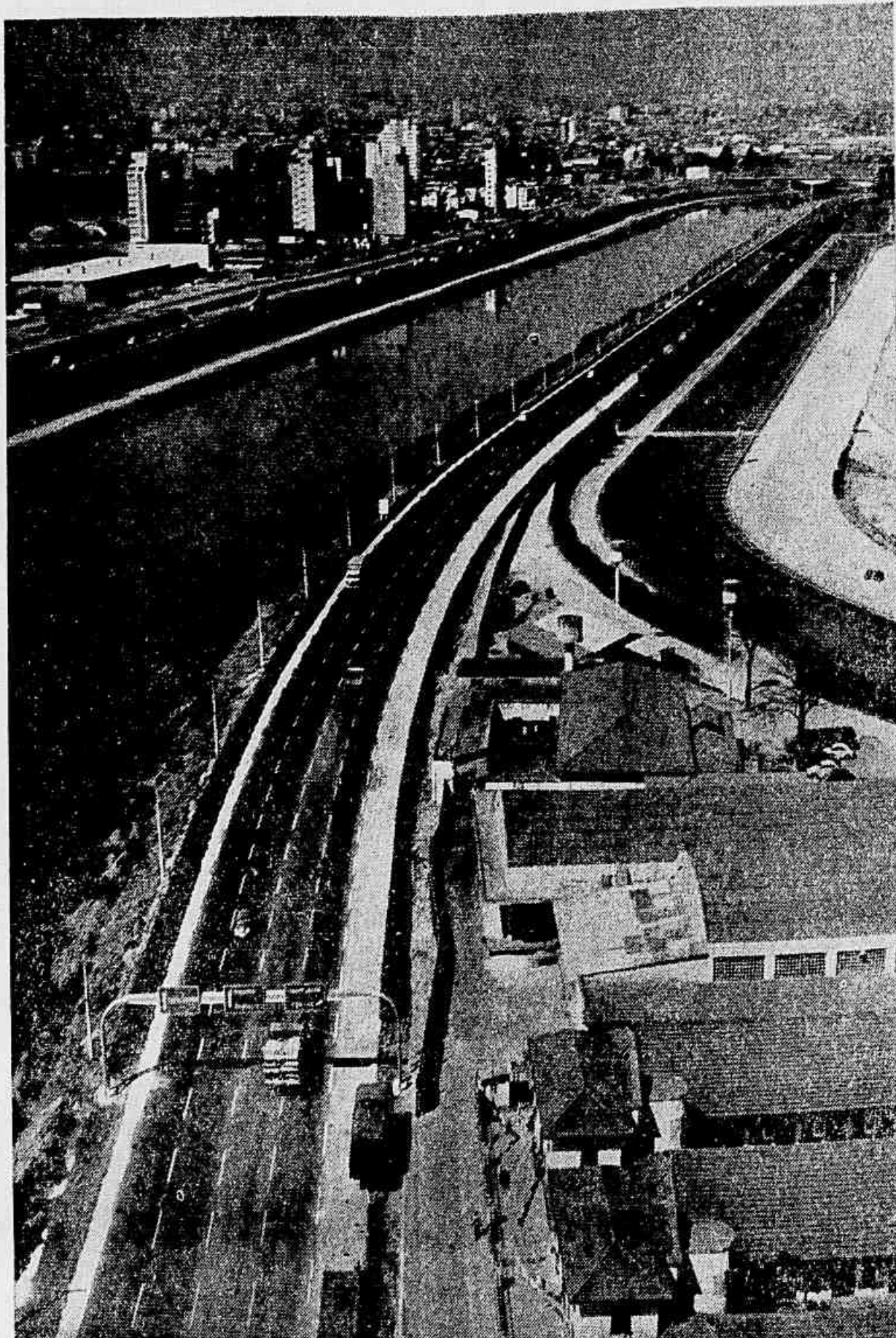
Foto aérea do Anel Rodoviário, próximo ao hipódromo da Cidade Jardim, vendo-se o moderno sistema de sinalização ali implantado.
