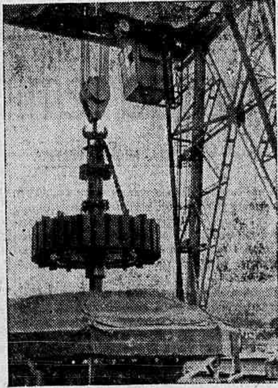
ITUTINGA — Vista da montagem do rotor da primeira unidade. Situada entre as importantes cidades mineiras de São João del Rei e Lavras, a usina de Itutinga terá a capacidade final de 60.000 HP. A construção da usina ficou a cargo da Cia. de Eletricidade do Alto Rio Grande, subsidiária da CEMIG e compreende todas as obras civis para a potência final. Já estão instaladas inicialmente duas unidades de 17.000 HP cada.
