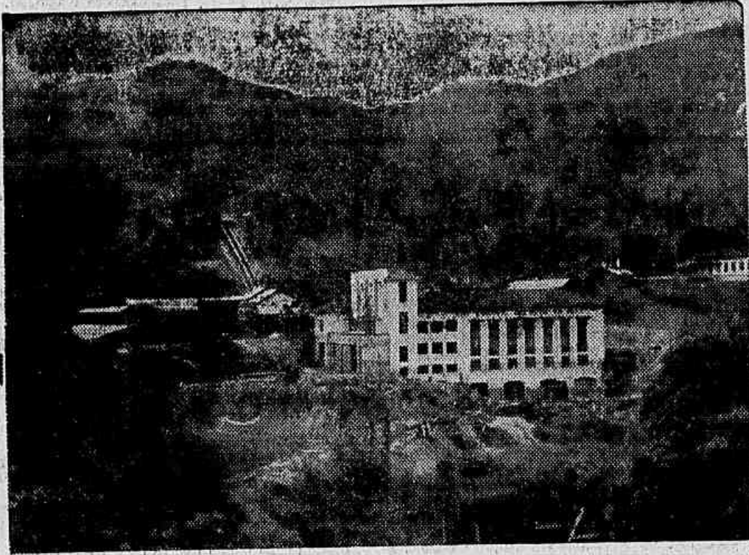
PIAU — Vista geral da usina. Destinada a abastecer a importante região de Santos Dumont, Juiz de Fora e Barbacena, a usina terá a capacidade final de 37.500 HP, em três unidades geradoras de 12.500 HP cada uma. Duas dessas unidades entram agora em funcionamento. A obra esteve a cargo da Central Elétrica do Piáu, subsidiária da CEMIG.
