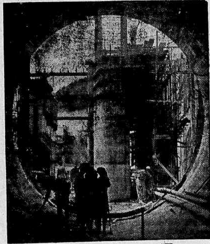
SALTO GRANDE — A usina do Salto Grande é o principal dos projetos em execução no Estado de Minas Gerais. A sua construção, a cargo da Cia. de Eletricidade do Alto Rio Doce, subsidiária da CEMIG, inclui o desvio das águas do Rio Santa Antônio, por um túnel de 3.200 metros de extensão, até o rio Guanhães. Daí, por um outro túnel de 4.400 metros de comprimento, as águas vão ter à casa de força, com capacidade de 140.000 HP. Estão em montagem duas unidades de 35.000 HP, cada uma e já em fabricação as duas demais.
