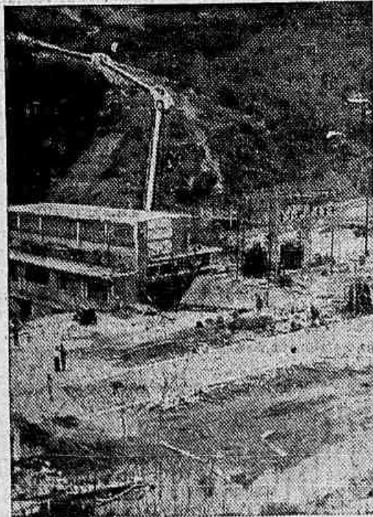
TRONQUEIRAS — Vista de conjunto da usina. O sistema completo de energia da região de Governador Valadares está a cargo da Cia. de Eletricidade do Médio Rio Doce, subsidiária da CEMIG. A capacidade final da usina será de 12.000 HP. Aham-se instalados inicialmente dois grupos de 3.000 HP cada um. A rede de transmissão, de 45 quilômetros de extensão, transporta a energia para Governador Valadares, na tensão de 33.000 volts. A rede de distribuição de 11.500 volts é a mais moderna do Estado.
