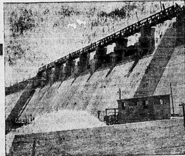
CAJURU — Vista da barragem de regularização, situada 20 quilômetros a montante da usina do Gafanhoto, que serve à cidade Industrial de Belo Horizonte. Esta barragem, que se destina a regularizar a vazão do rio Pará, permitindo a plena utilização da potência instalada naquela usina, tem o comprimento total de 438 metros, dos quais 341 em concreto, e armazena 190 milhões de metros cúbicos de água. Esta obra faz parte do plano de regularização do regime fluvial do rio São Francisco e foi, em parte, custeada pela Comissão do Vale do São Francisco, tendo sua construção ficado a cargo da CEMIG.
